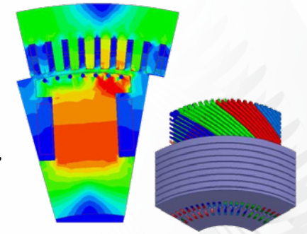
ANSYS Maxwell simulation
